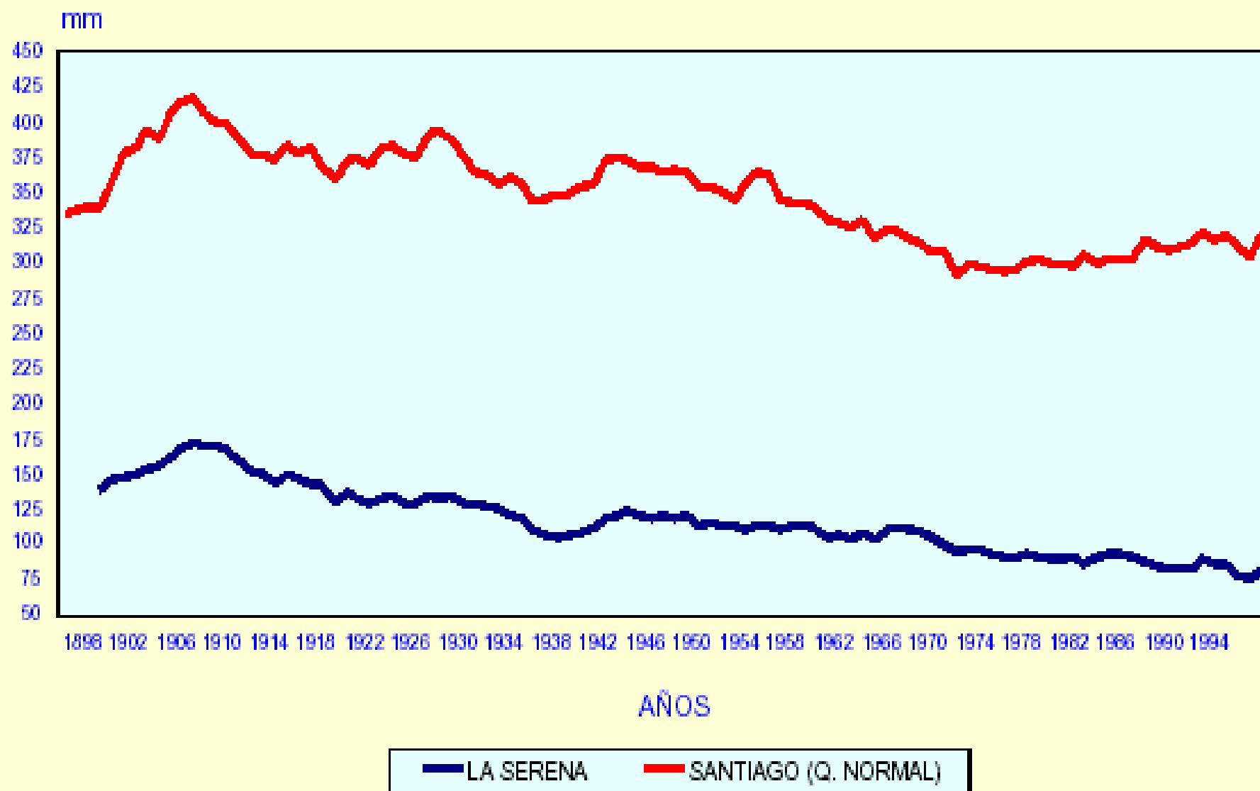
Figura 6. Precipitaciones Promedios Móviles cada 30 años
